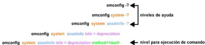
Figura 2-1. Distintos niveles de ayuda para un comando
